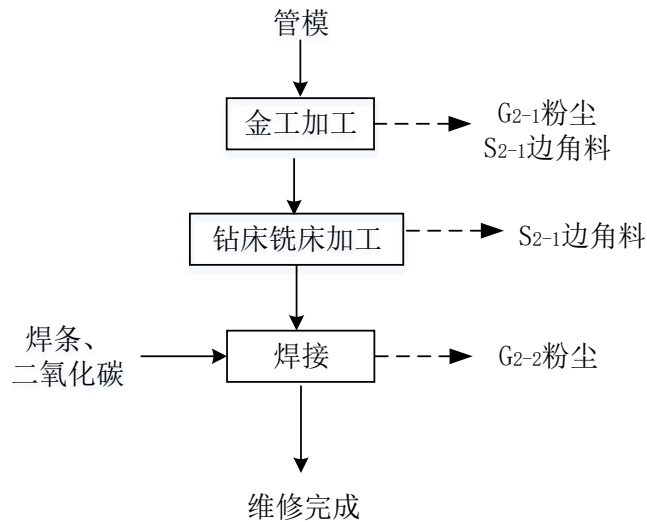
图 1-9 管模维修工艺流程及产污环节图
