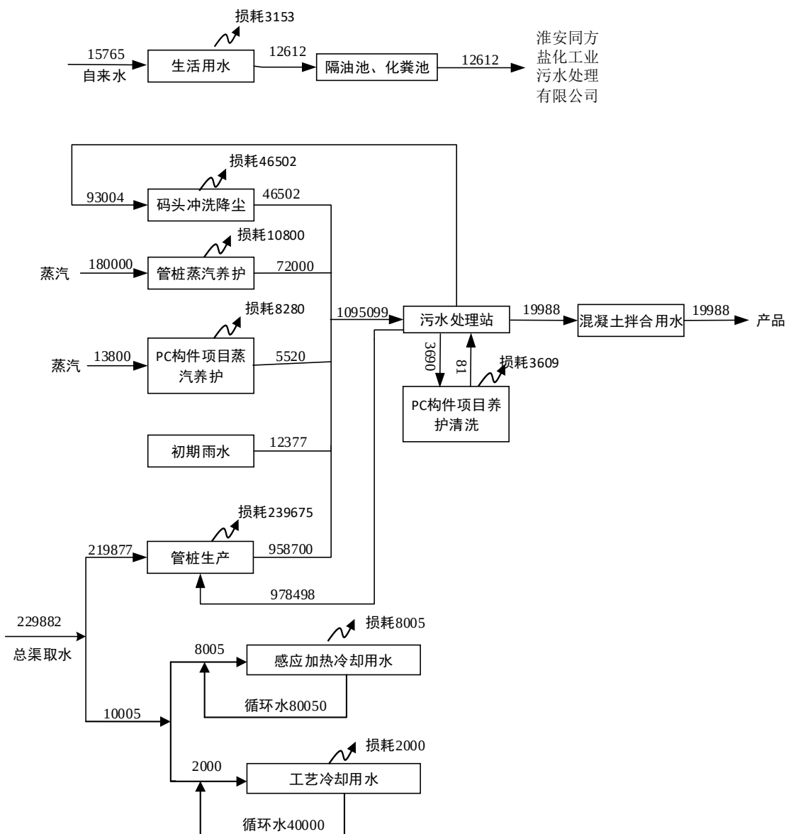
图 5-2 项目建成后全厂给排水平衡图 (m³/a)
