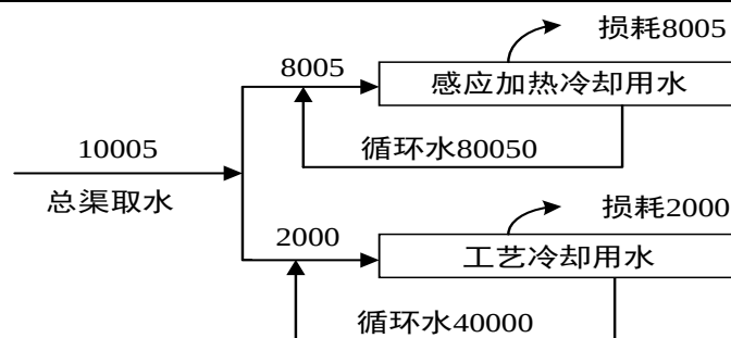
图 5-1 建设项目给排水平衡图 (m³/a)
