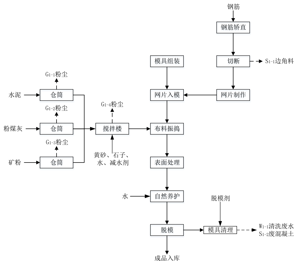
图 1-6 PC 构件生产工艺流程及产污环节图
