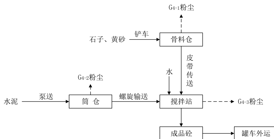
图 1-4 商品混凝土生产工艺流程及产污环节图
