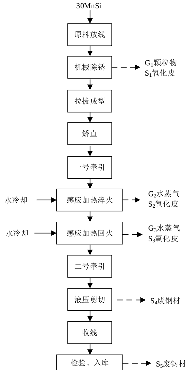
图 5-1 PC 钢棒生产工艺流程及产污环节图
